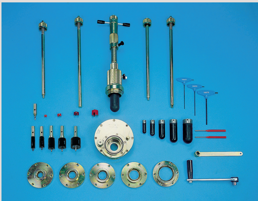
Proco Services blockeringsutrustning Ministop ¾" – 2", anpassad för Cu22 till DN50.
